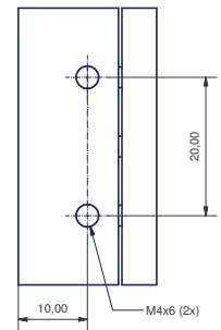
Halteblock LED-Kopf HP
